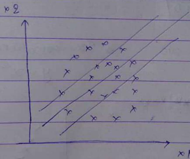
Linear SVC
