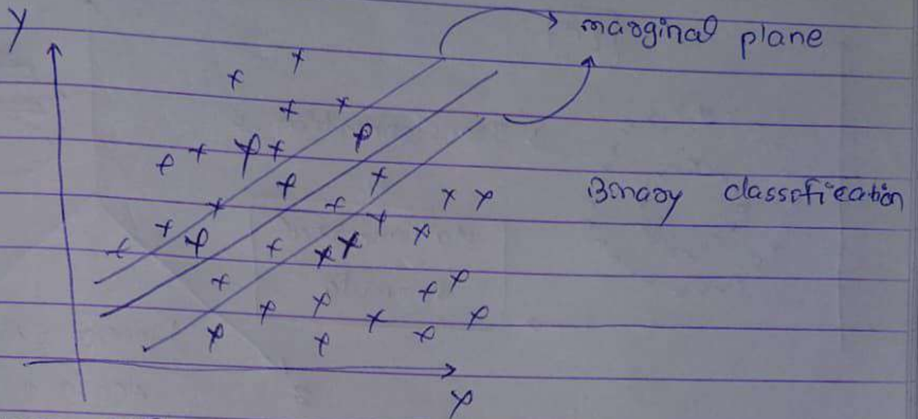
Linear SVC
